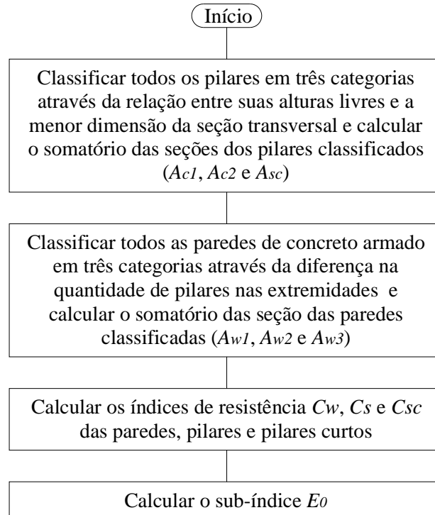
Figura 17 – Fluxograma para cálculo do sub-índice E_0 no primeiro nível de avaliação (Adaptada de Hirosawa:1992)
