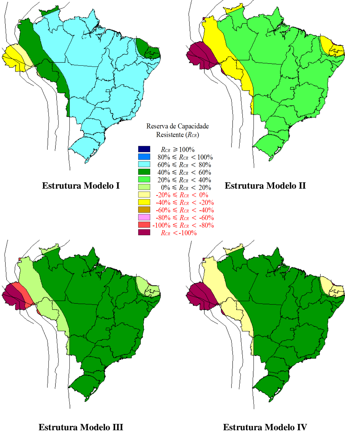
Figura 53 - Mapas de vulnerabilidade sísmica das estruturas modelo – Terreno Classe E
