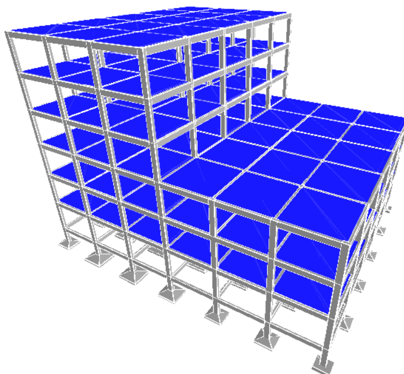
Figura 42 - Pórtico da Estrutura Modelo IV
