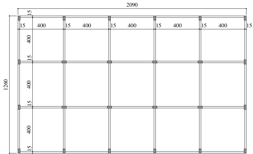
Forma do pavimento Nível +11,20
