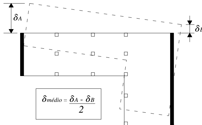
Figura 13 - Irregularidade torsional (SEI7/ASCE:2005)
