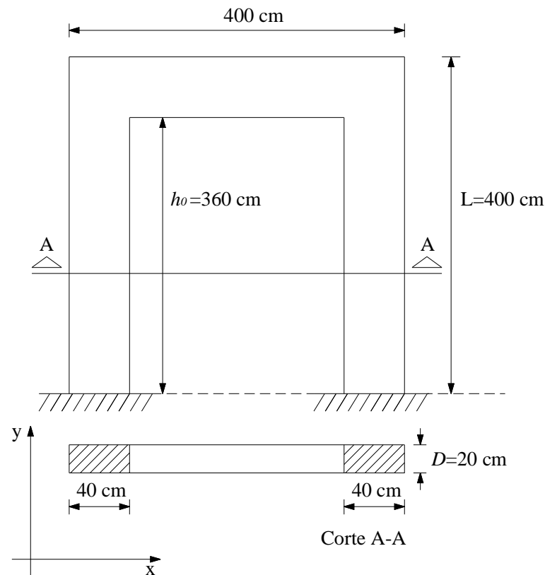
Figura 23 – Pórtico em concreto armado
