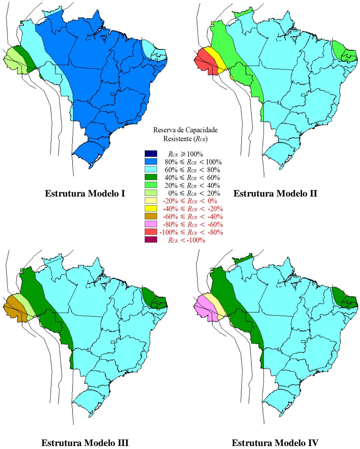
Figura 51 - Mapas de vulnerabilidade sísmica das estruturas modelo – Terreno Classe C
