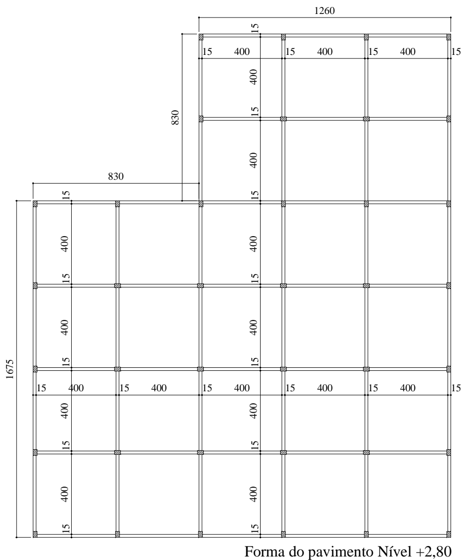
Figura 31 – Planta de forma do nível +2,80 da Estrutura Modelo II
