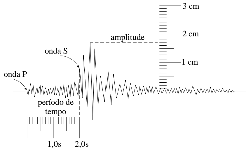
Figura 1 - Leitura de amplitude em sismômetro (Adaptada Lindeburg e McMullin:2008)
