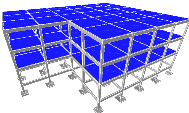
Figura 30 - Pórtico da Estrutura Modelo II
