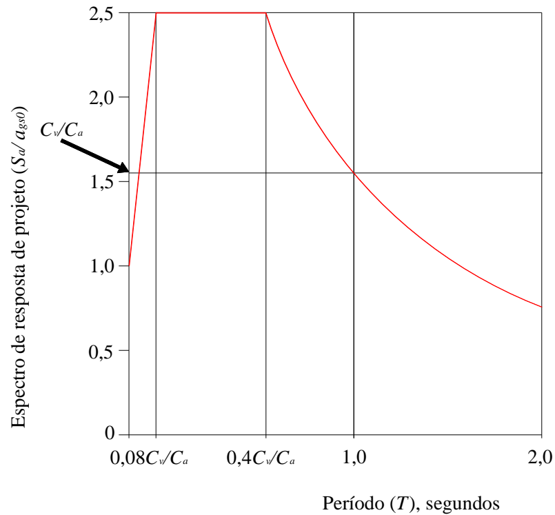
Figura 10 – Espectro de resposta de projeto (NBR 15421:2006)
