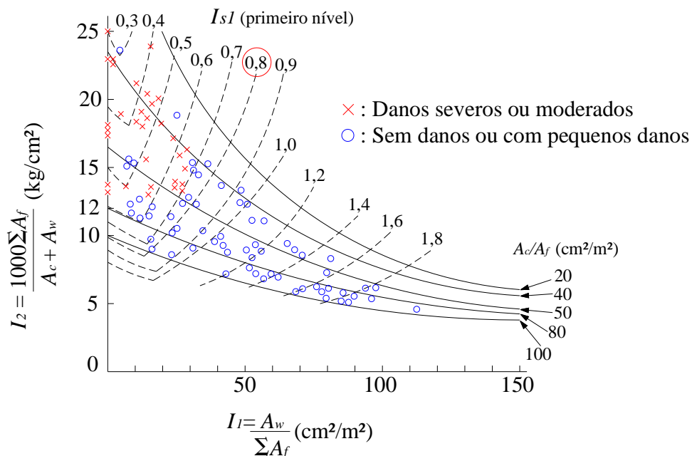
Figura 21 – Relação entre I_s e a severidade dos danos verificados (Adaptada de Unemura:1980)
