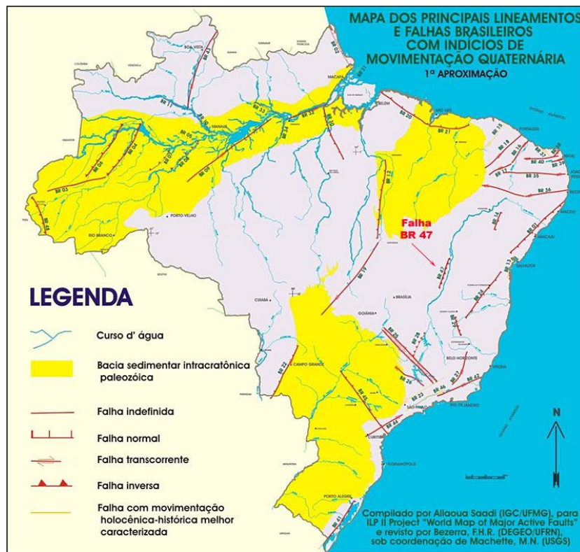
Figura 5 - Mapa das principais falhas tectônicas brasileiras (Saadi:2002)
